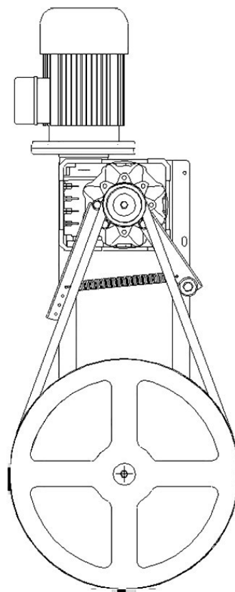
Рабочее положение натяжителя
