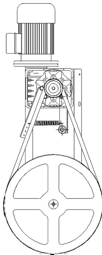
Транспортное положение натяжителя
